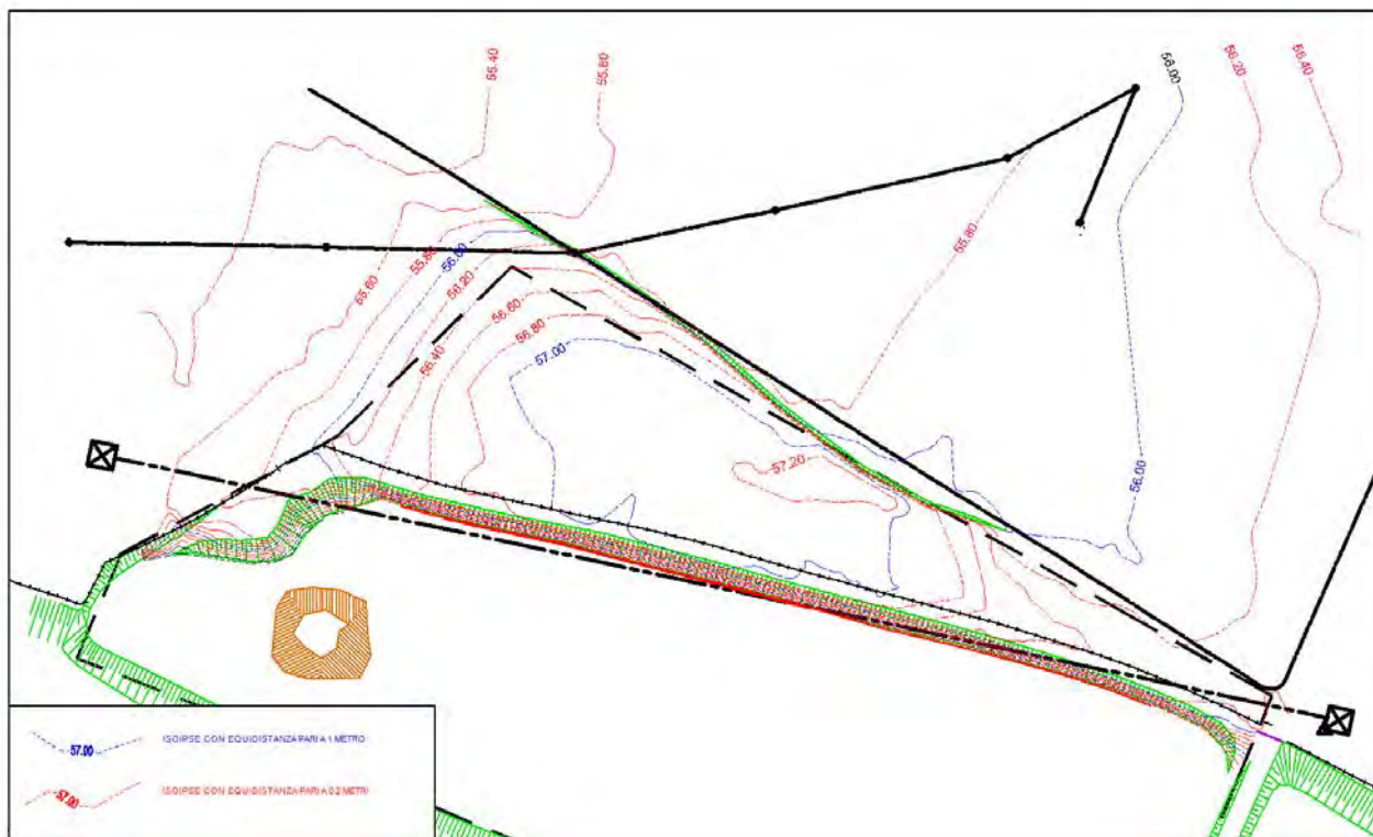
Fig. 26 – Cartografia delle isoipse dello stato di fatto
