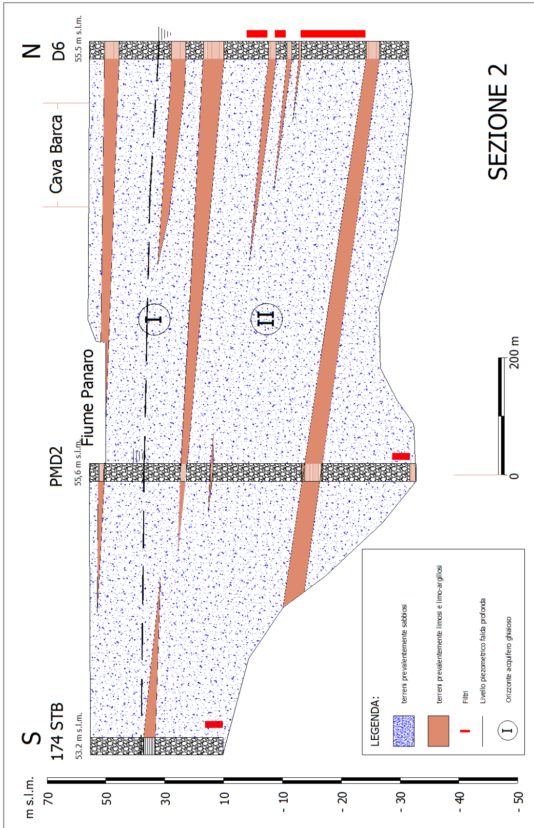
Fig. 50 – Sezione idrogeologica 2
