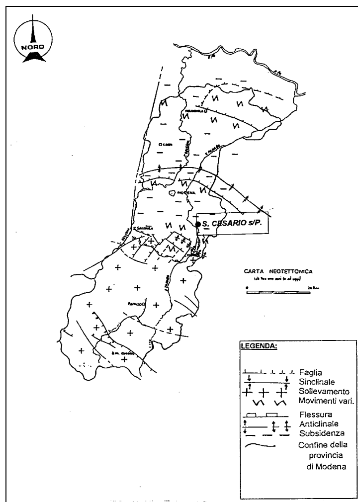
Figura 19 – Neotettonica
