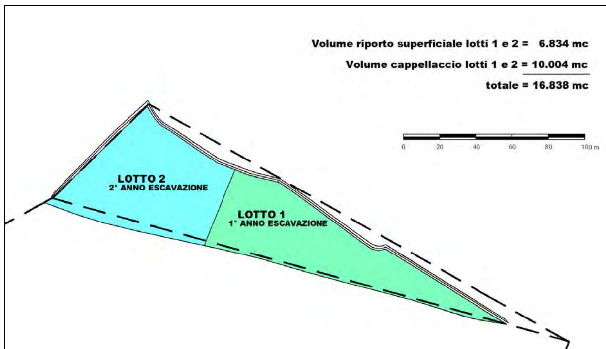
Fig. 36 - Volumi riporto superficiale e terreni di cappellaccio
